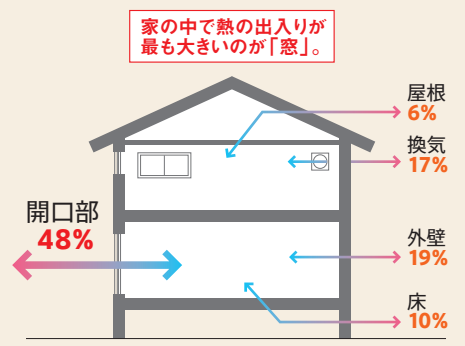
出典:(社)日本建材産業協 省エネルギー-建材普及センター 「21世紀の住宅には、開口部の断熱を...」より 平成4年省エネ基準で建てた住宅モデルにおける例
